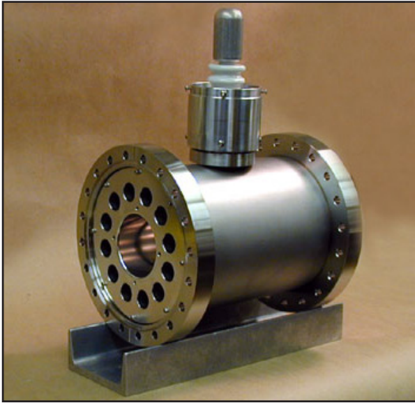
NEC Einzel Lens with CF flanges
